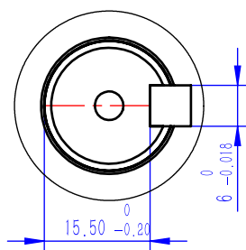
轴端带键尺寸图
